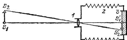
Рис. 244. Схема фотоаппарата: 1 — объектив, 2 — камера, 3 — фото-пленка
