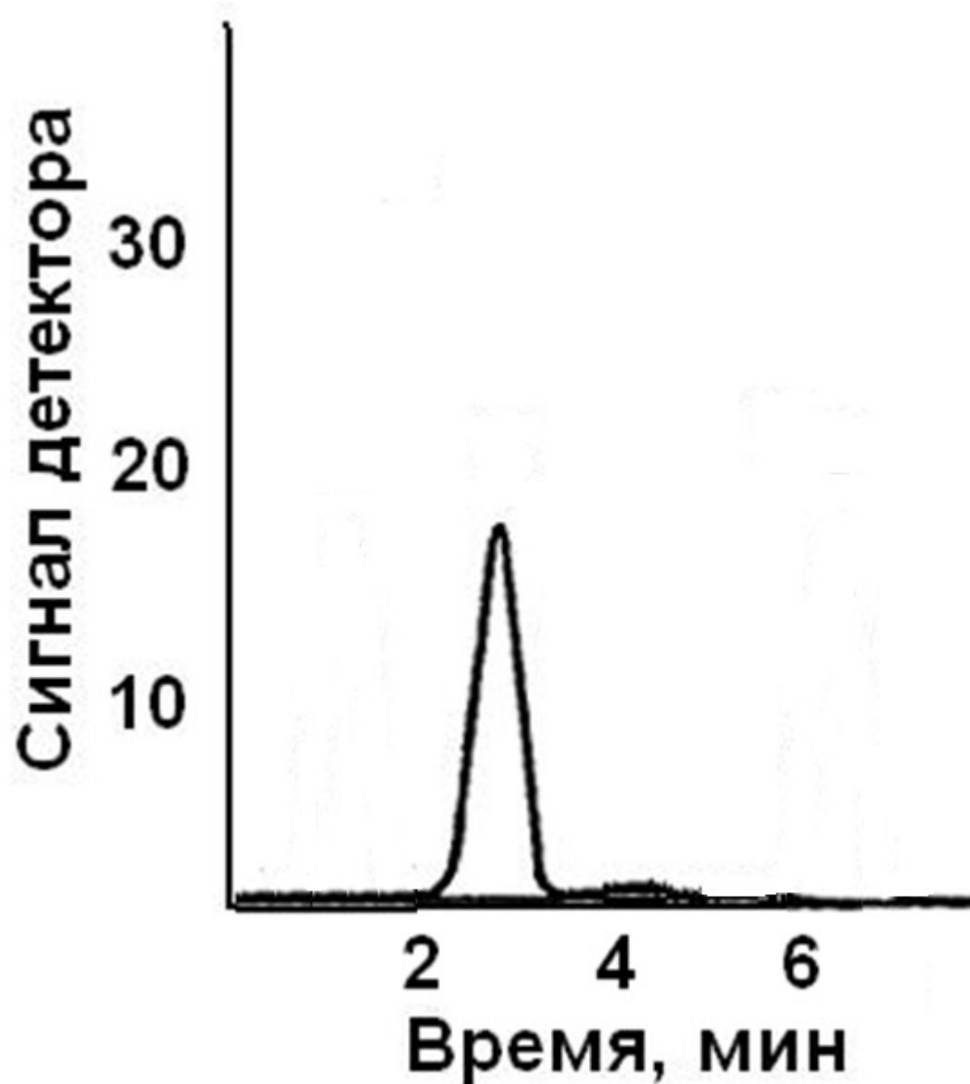
Хроматограмма метанола
