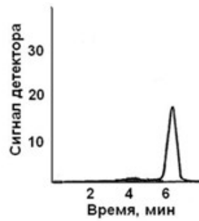
Хроматограмма этанола
