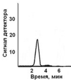
Хроматограмма метанола
