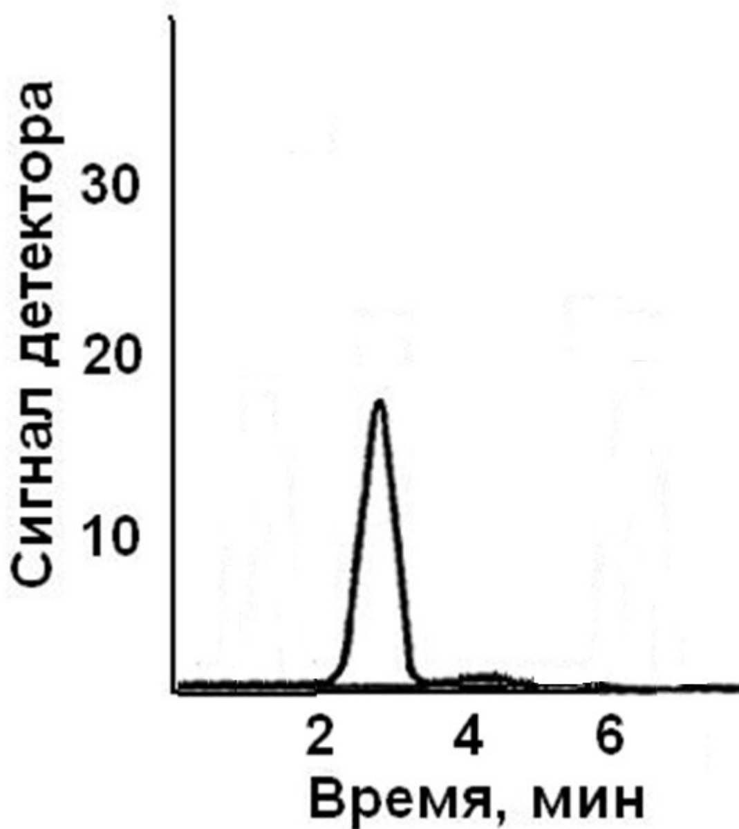
Хроматограмма метанола
